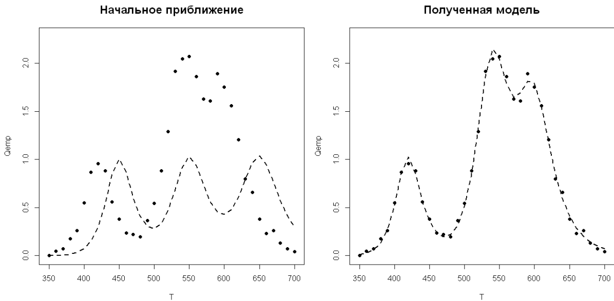
Рис. 1 – Результаты разложения спектра при правильном выборе числа компонент
