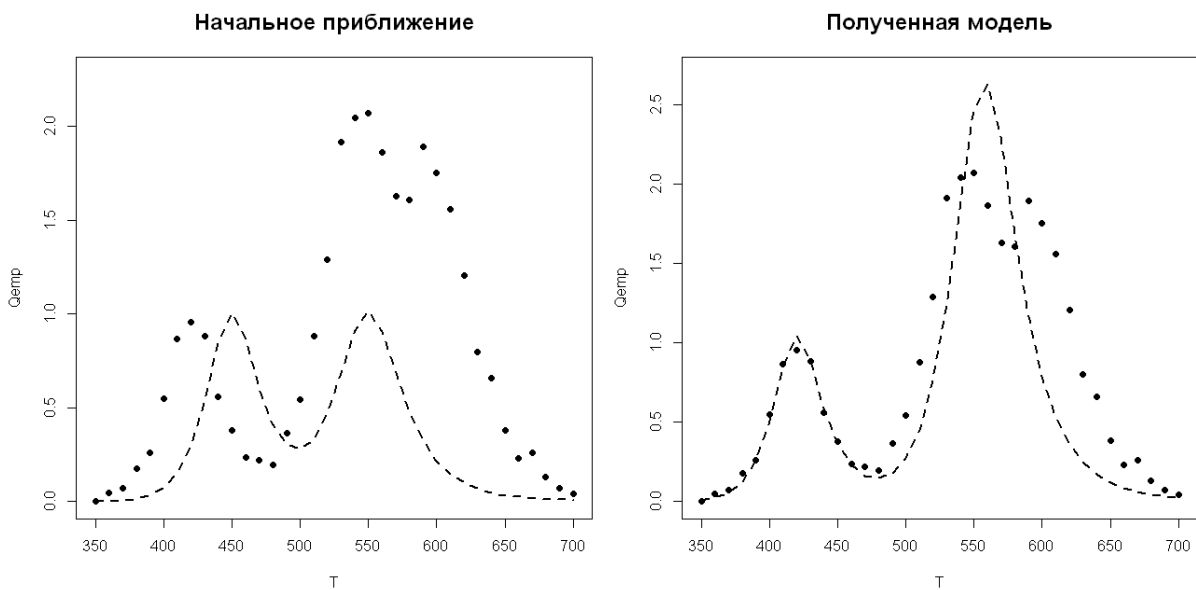
Рис. 2 – Результаты разложения спектра при ошибочном выборе числа компонент
